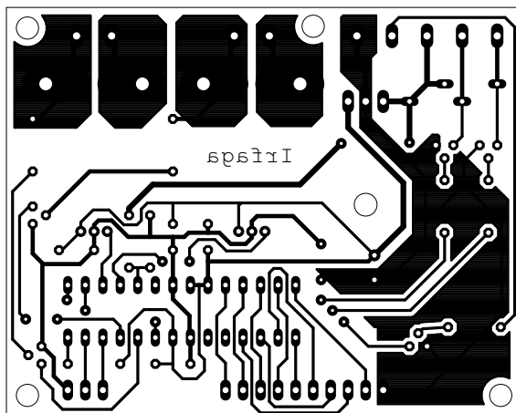
Nadzor svetala u automobilu
