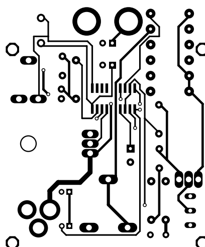
Zapper (desno - donji sloj - Bottom, levo - gornji sloj - Top)
