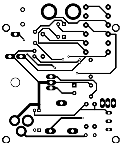
Zapper (desno - donji sloj - Bottom, levo - gornji sloj - Top)
