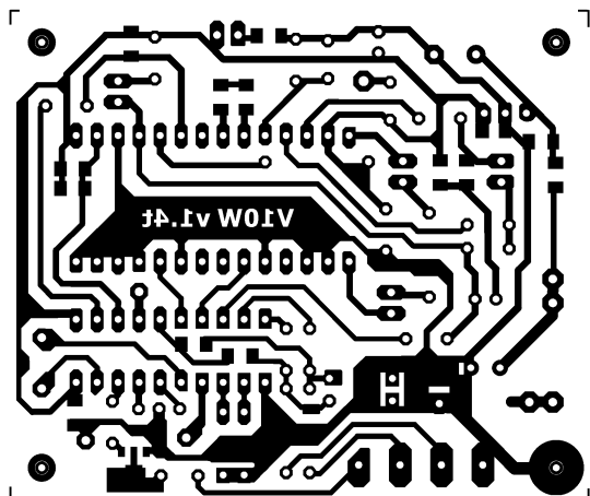
Uređaj za snimanje i reprodukciju kratkih govornih poruka
