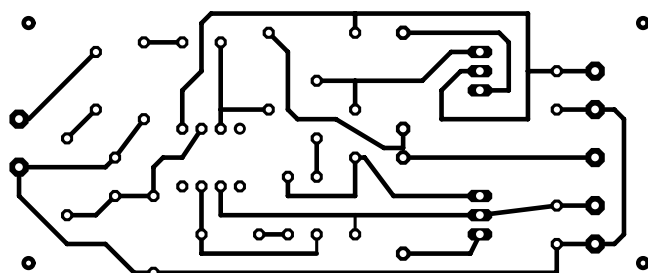
HiFi pojačavač za slušalice
