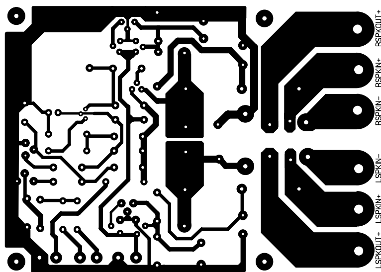
Univerzalna zaštita zvučnika i modul "mute"
