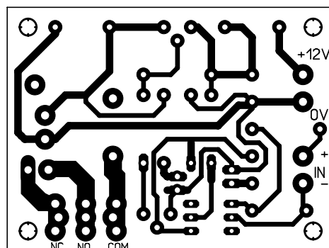
Jednosmerni relejni prekidač
