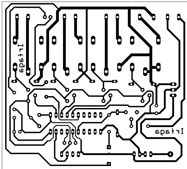
Alarm za automobil
