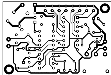
Prstenasti blic od LE dioda
