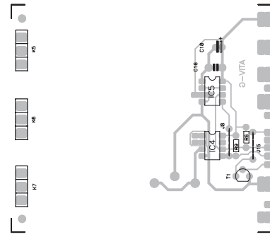
Akviziter - Nacrt montazne pločice - zadnja (Umanjeno 50 %)
