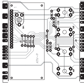
Akviziter - Nacrt montazne pločice - komandna tabla (Umanjeno 50 %)
