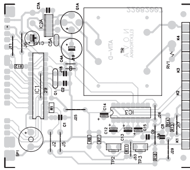
Akviziter - Nacrt montazne pločice - glavna (Umanjeno 50 %)
