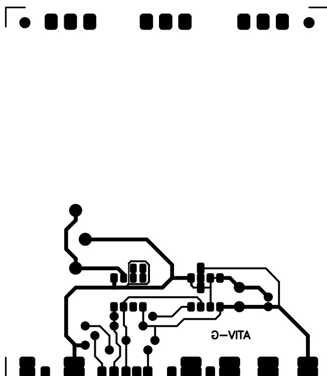
Akviziter - Nacrt montazne pločice
