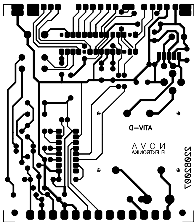
Akviziter - Nacrt pločice - glavna
