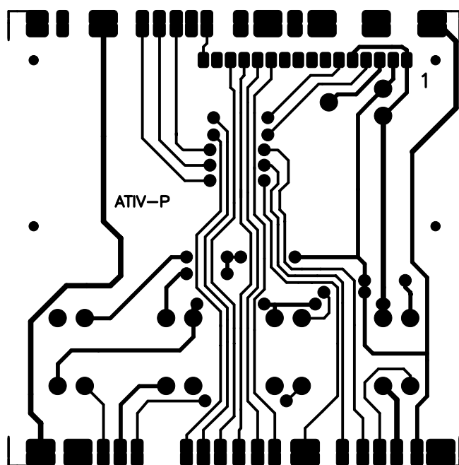
Akviziter - Nacrt pločice - komandna tabla
