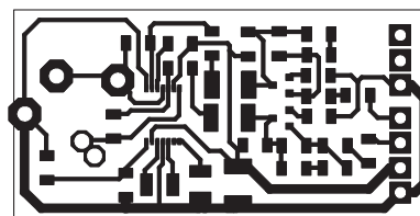
Pojačavač sa 3D zvukom za slušalice
