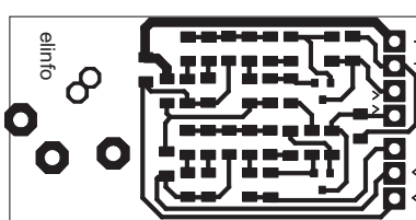
Visokonaponsko napajanje - inverter
