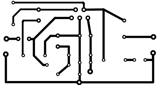
Pojačavač sa TDA2040
