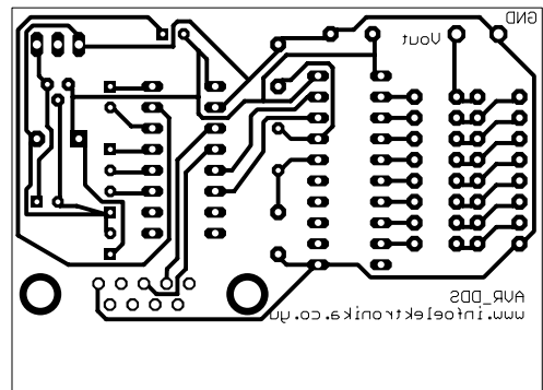
Generator funkcija sa digitalnom sintezom
