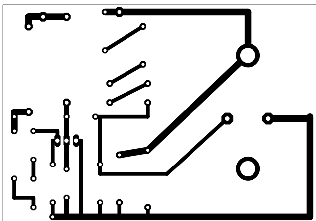
Tranzistorsko paljenje za Yugo-45
