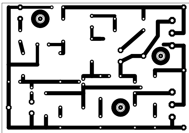
Pojačavač u A klasi
