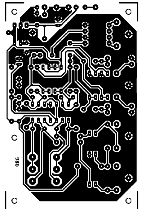
Stereo mikrofoni za zvučne karte
