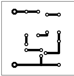
Punjač akumulatora - indikator napunjenosti
