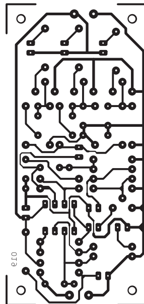
Konvertor zvuka u svetlost (članak iz prethodnog broja)
