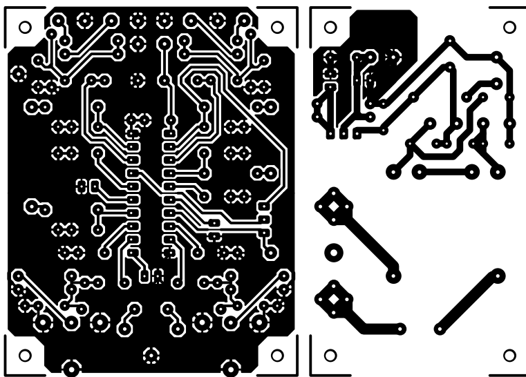
Kontrola zvuka pomoću jednog čipa
