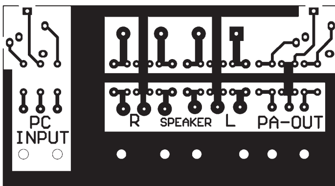
Univerzalno PC audio pojačalo, terminal panel, lemljena strana
