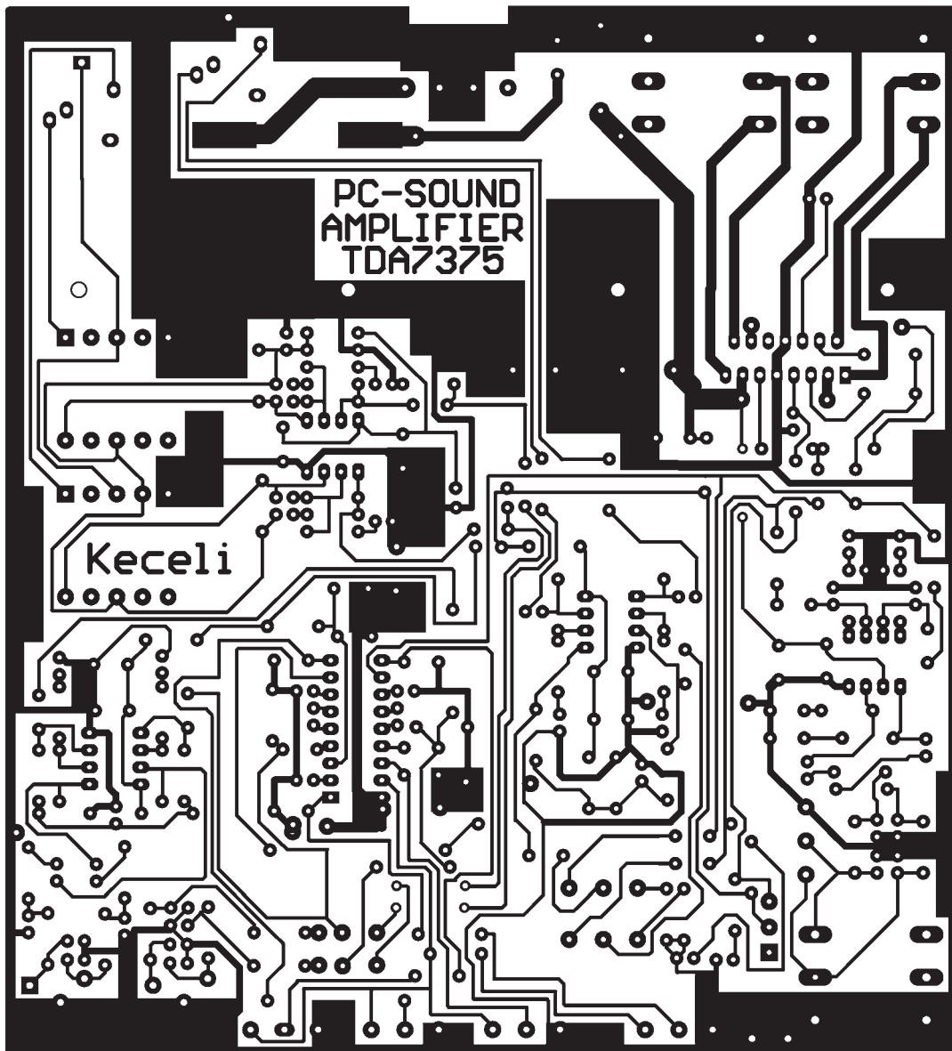
Univerzalno PC audio pojačalo, panel pojačala, lemljena strana
