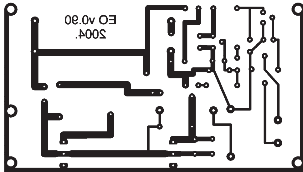
Elektronski mrežni osigurač sa podesivim pragom okidanja
