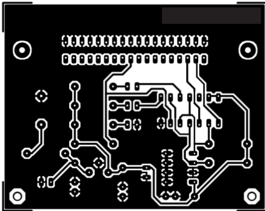
Jednostavan EEPROM programator
