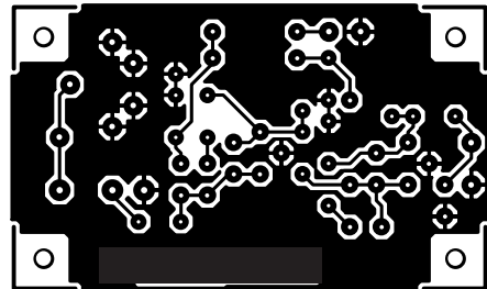
Pobuđivač za kablovski radio
