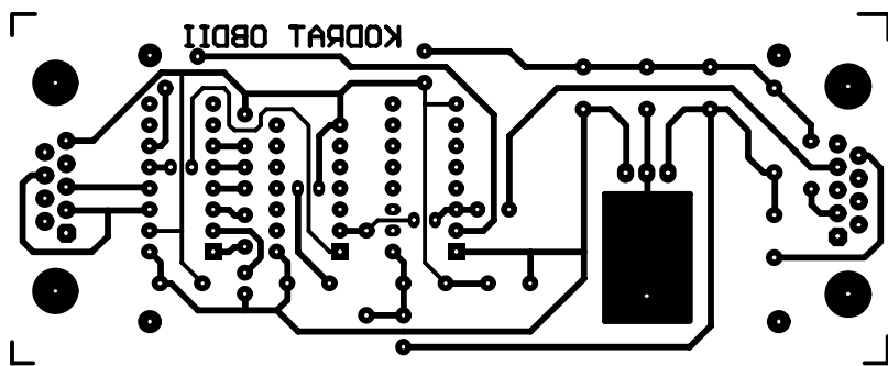
Jednostavan OBD-2 interfejs za dijagnostiku automobila
