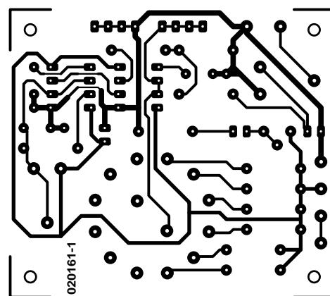
Merač kapaciteta
