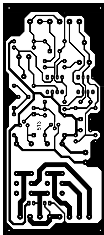
Sklop za horizontalno zakretanje solarnih panela
